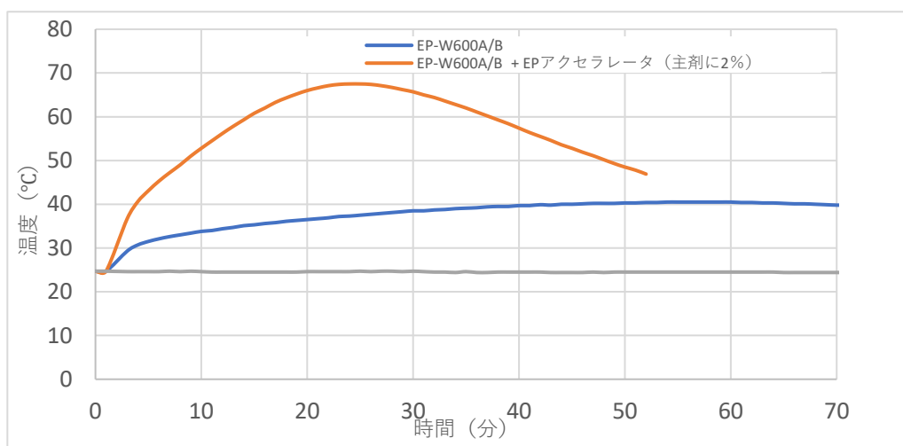
【使用例】「アルファレジン EP-W600A/B」に EP アクセラレータを添加した時の硬化発熱曲線 (100g スケール)
